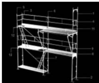
Andamio Europeo
